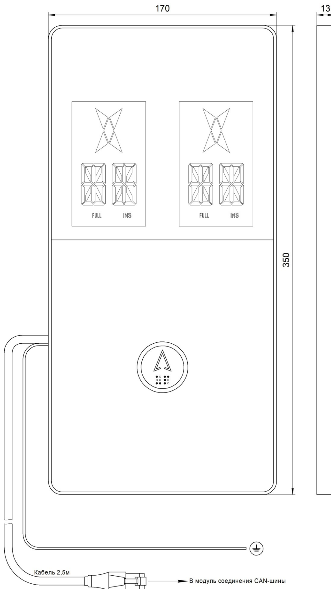
Рис.1 Внешний вид, габаритные и установочные размеры Вызывного поста МАЛАХИТ (жгут RJ45) НШЕК.468381.101
